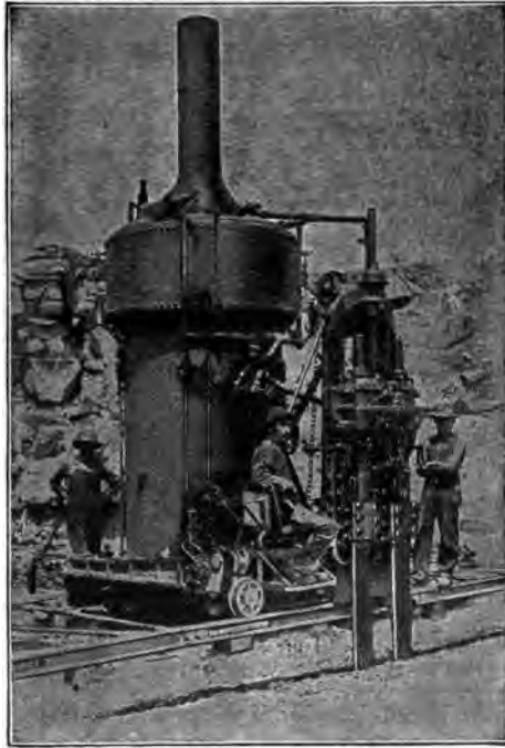
Fig. 124. Duplex Channeler.
